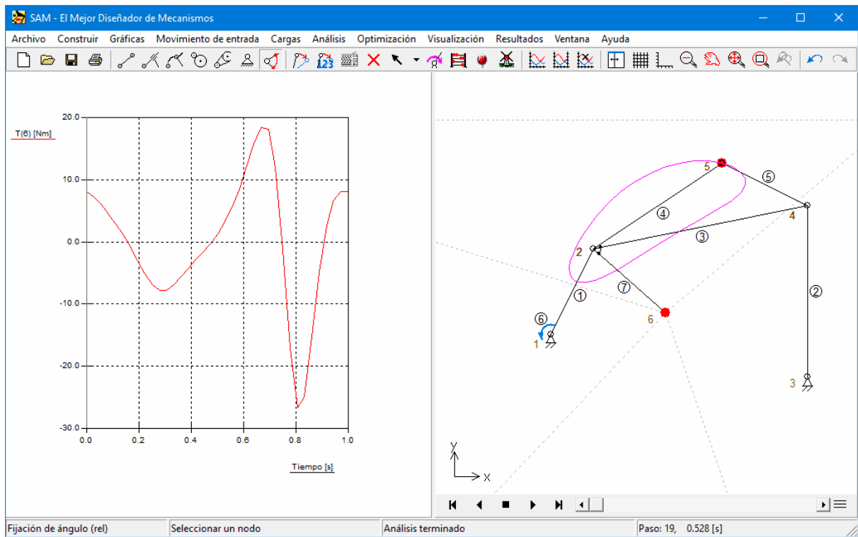
Elemento 7 incluida la masa de compensación agregado
