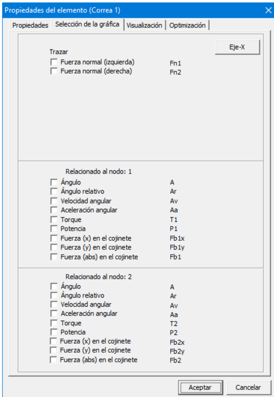
Propiedades calculables del elemento correa
