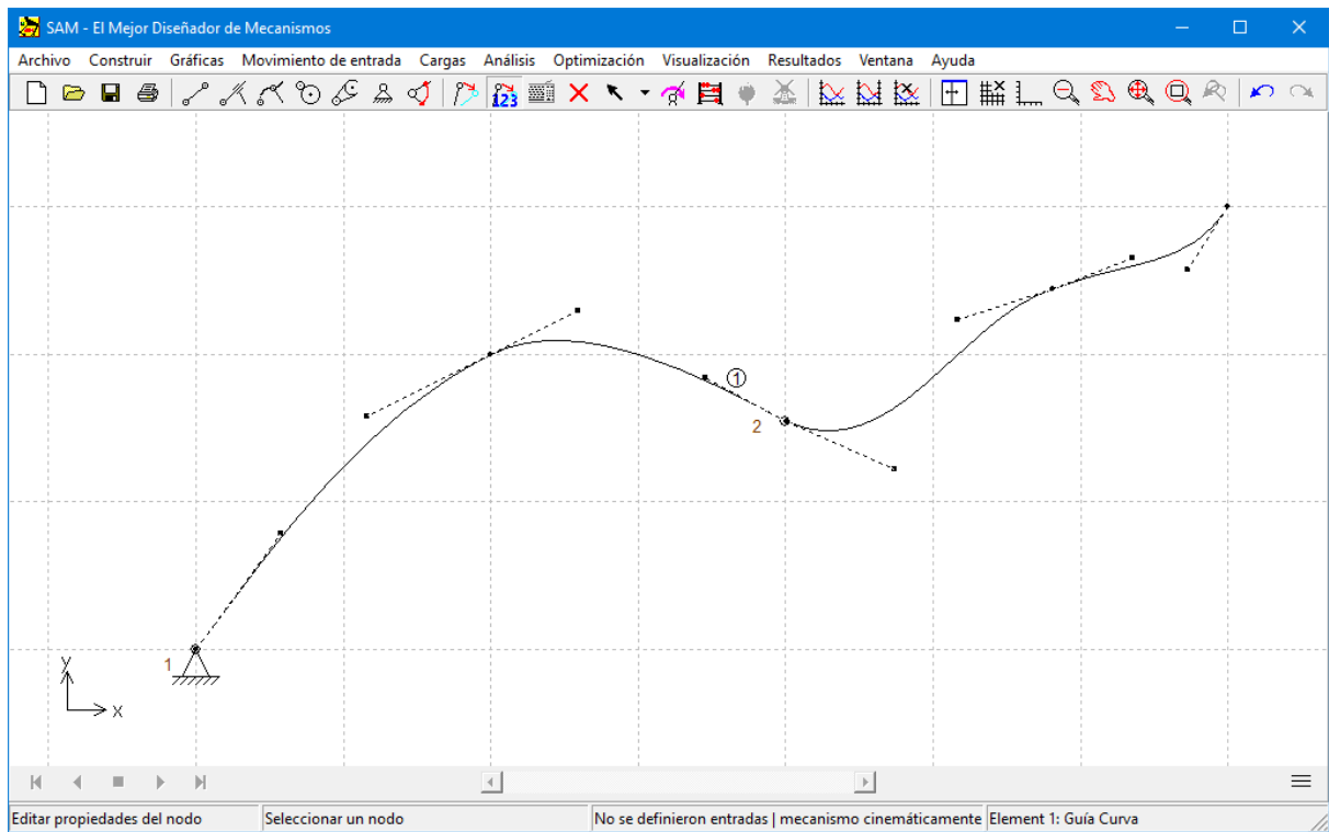
La definición de guía curva se basa en puntos Bézier
