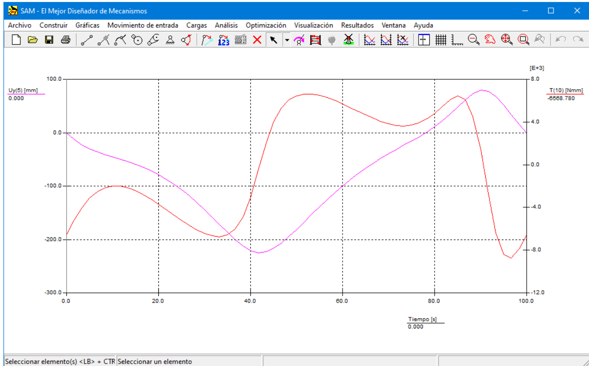
Enlace de transferencia de la posición vertical & torque motor estático
