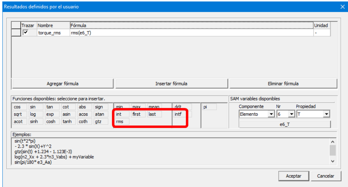
Captura de pantalla que muestra las nuevas funciones rms, first, last e intf
