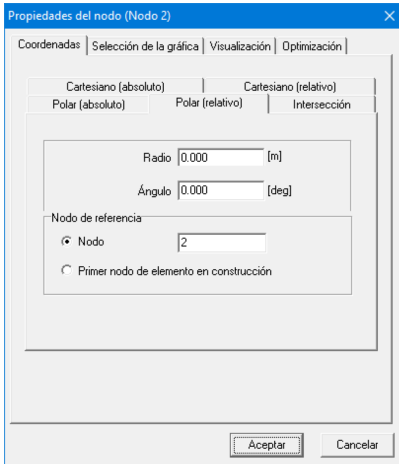
Cuadro de diálogo para la "Construcción" de coordenadas nodales exactas
