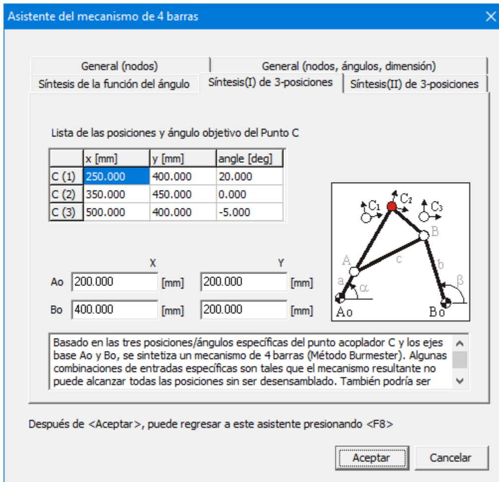
Asistente del Mecanismo de 4 barras: Síntesis (I) de 3 posiciones
