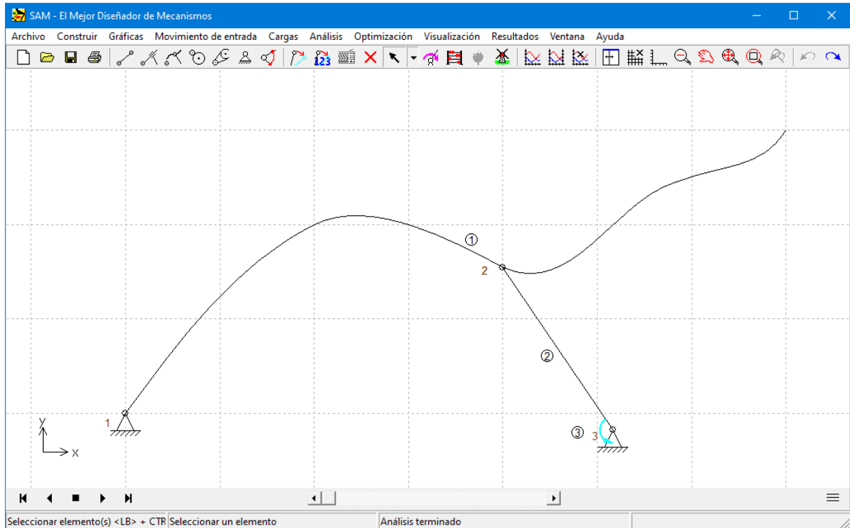
Ejemplo de un elemento guía curva (1) combinado con una manivela y un motor
