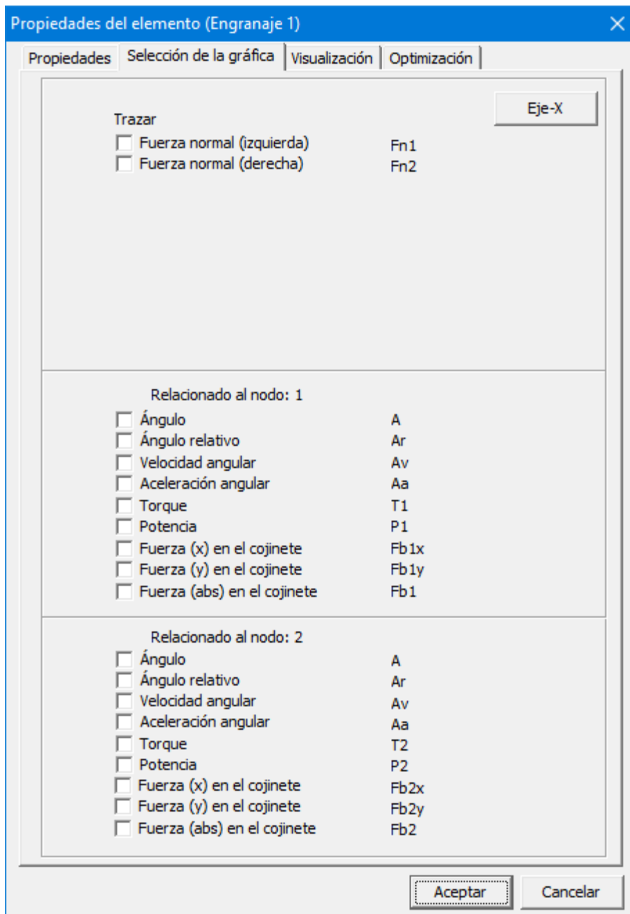
Propiedades calculables del elemento engranaje
