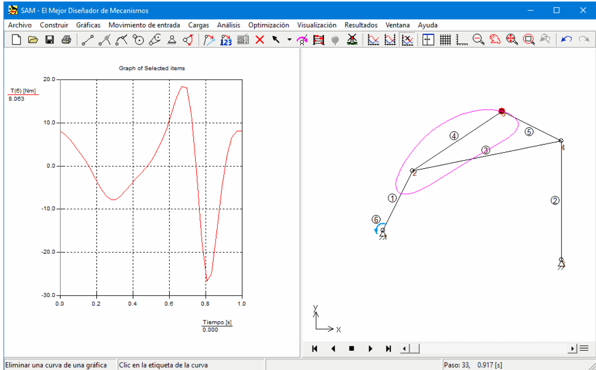
Mecanismo de referencia (a. torque motor b. mecanismo y trayectoria del punto acoplador)
