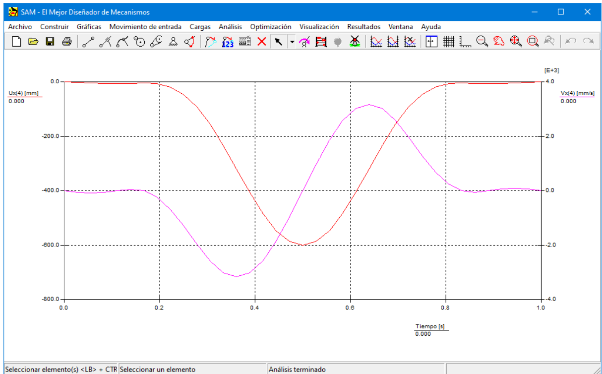
Desplazamiento y Velocidad de Salida del Mecanismo Hipo-cíclico
