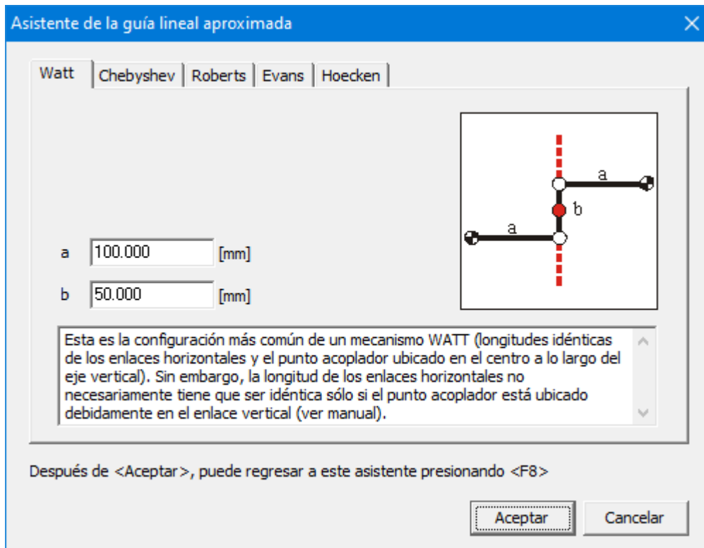
Asistente de movimiento de Línea Recta Aproximada: Watt
