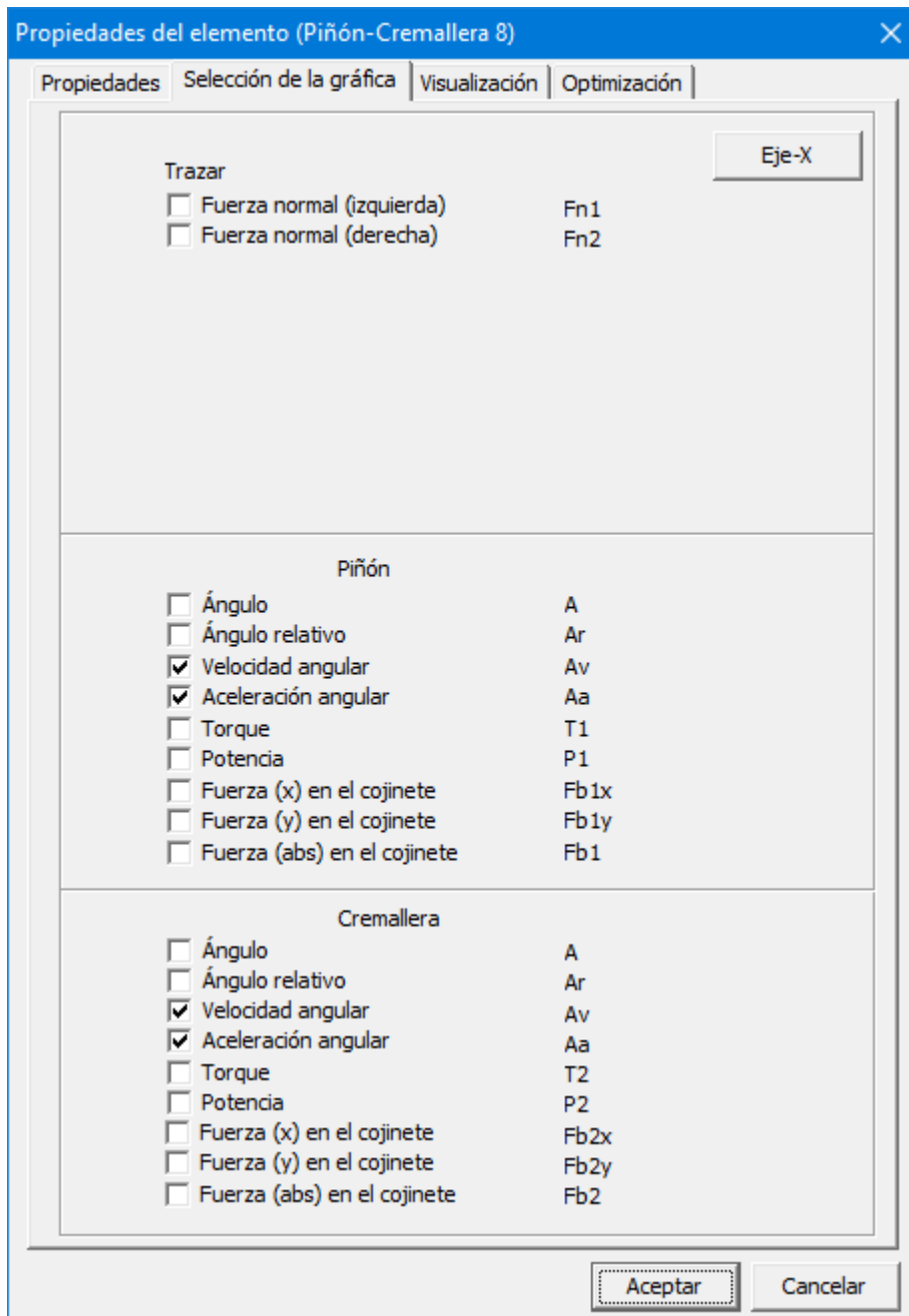
Propiedades calculables del elemento de piñón de cremallera
