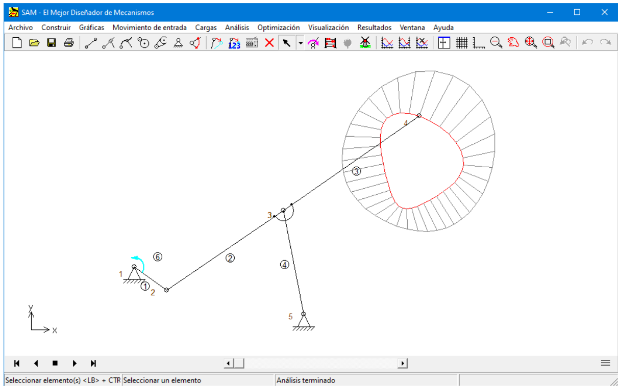
Mecanismo Balancín de Manivela (CRRK.SAM)
